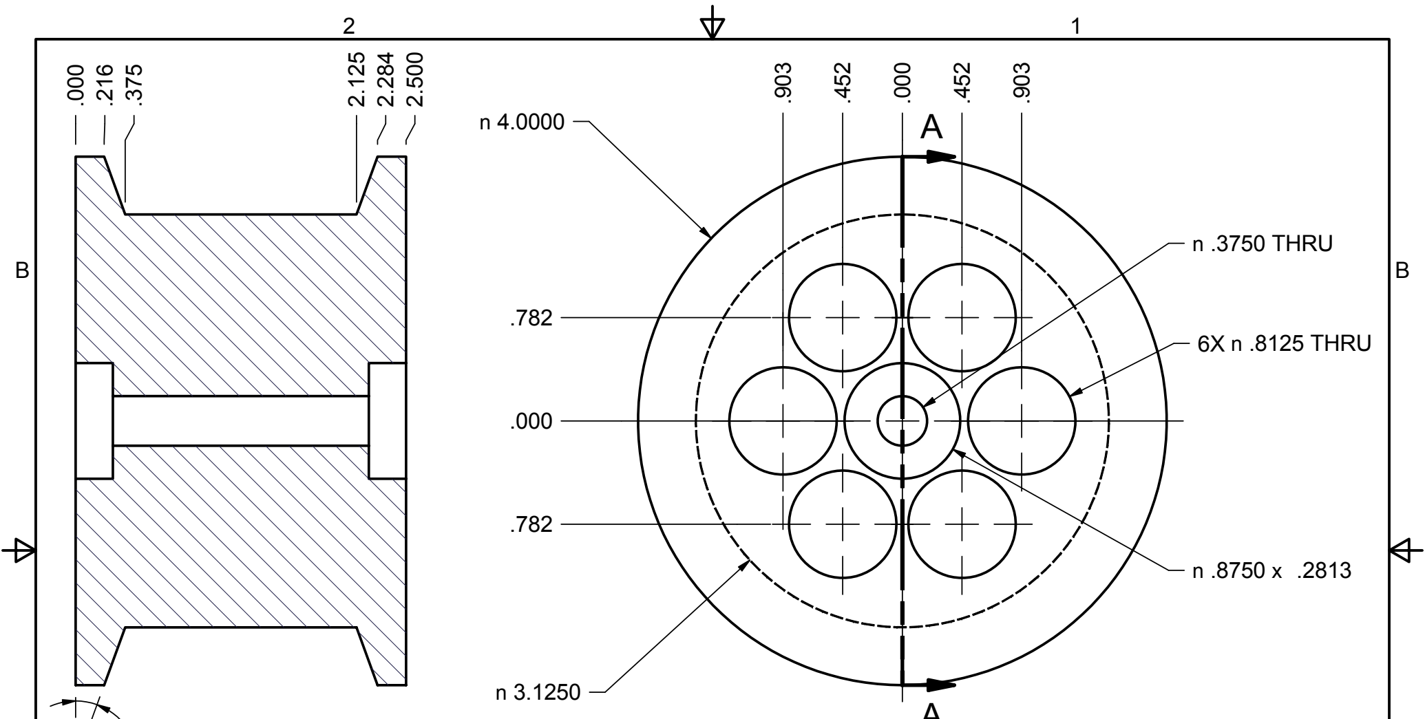
SECTION A-A SCALE 1 : 1
